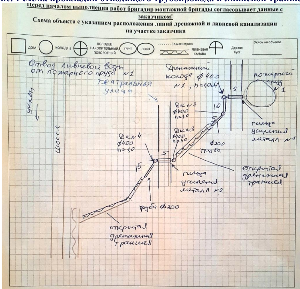
Рис. 2 Схема прокладки отводящего трубопровода и ливневой траншеи.
